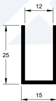
U-555 0,230 kg/m
