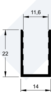
U-607 0,162 kg/m
