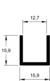
U-509 0,192 kg/m
