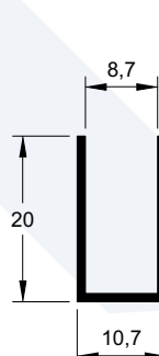
VT-727 0,130 kg/m
