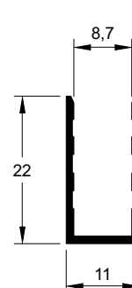
U-606 0,154 kg/m
