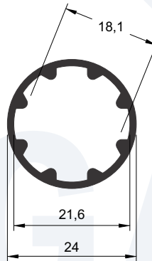
TM 1497 0,320 kg/m
