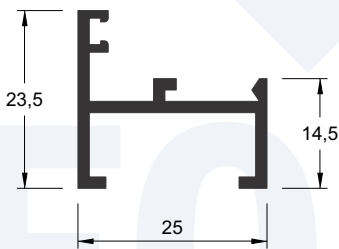
Y-197 0,298 kg/m
