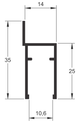
Y-106 0,222 kg/m
