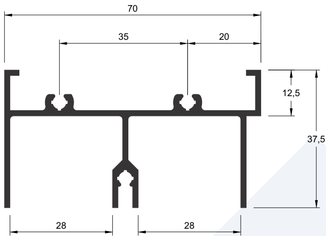
E-482 0,884 kg/m
