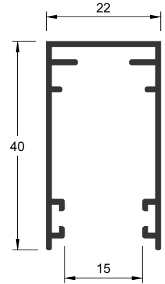
TM 1498 0,347 kg/m
