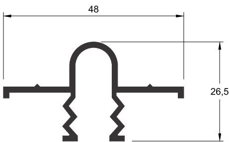
E-364 0,499 kg/m
