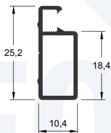
TM 1712 0,176 kg/m
