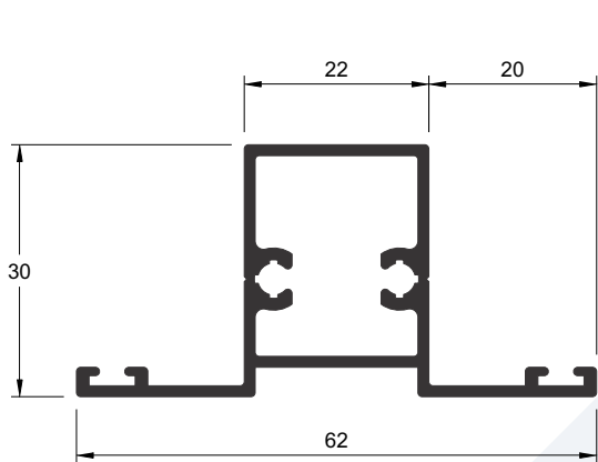
P-574 0,634 kg/m
