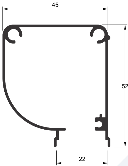
TM 1500 0,590 kg/m
