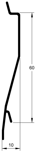
Z-201 0,250 kg/m
