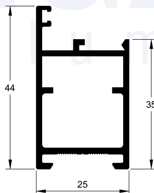
P-416 0,591 kg/m
