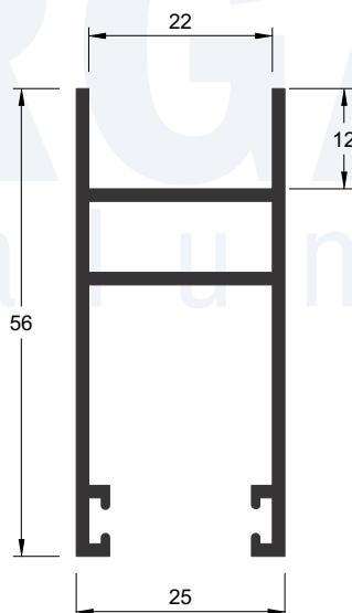
A-195 0,686 kg/m
