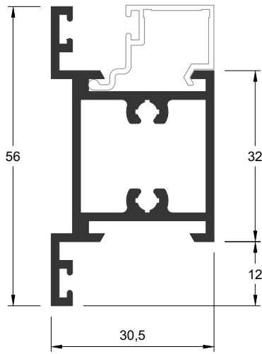
P-413 0,813 kg/m
