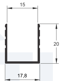
U-654 0,186 kg/m
