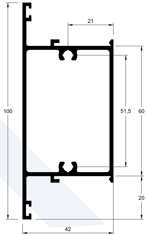
P-279 1,275 kg/m
