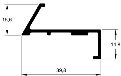
Z-033 0,350 kg/m
