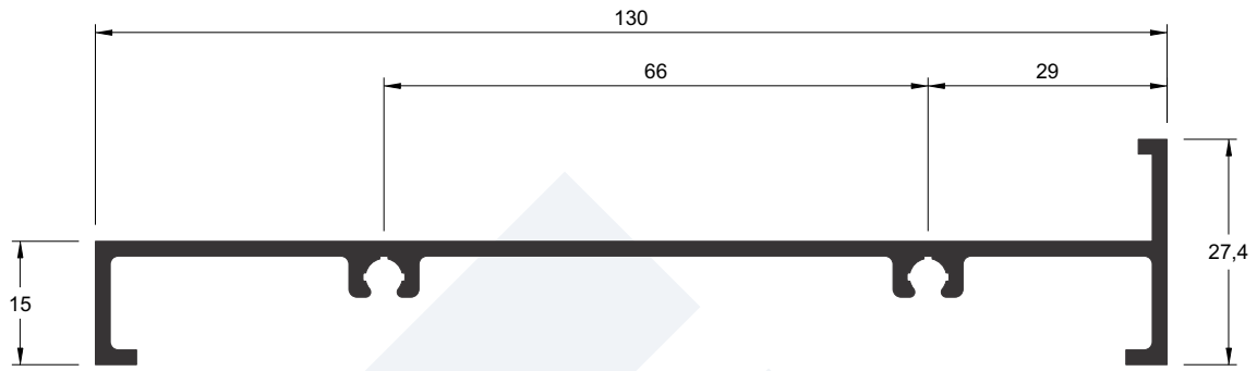
Y-350 0,984 kg/m
