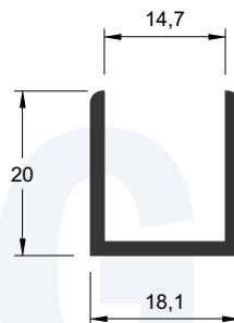
U-398 0,200 kg/m
