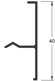
RA-006 0,168 kg/m
