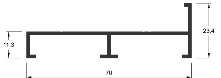
E-277 0,509 kg/m
