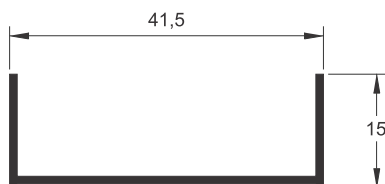
BXL-085 0,190 kg/m
