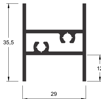
A-084 0,580 kg/m
