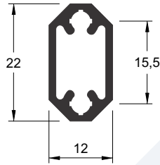
D-070 0,263 kg/m
