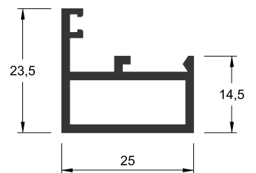
P-147 0,366 kg/m
