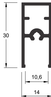
BX-040 0,316 kg/m
