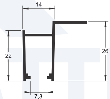
BXL-091 0,216 kg/m
