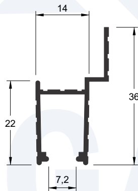
BX-088 0,203 kg/m
