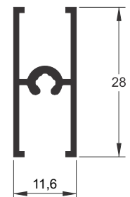
BXL-090 0,216 kg/m
