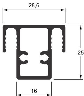
P-256 0,497 kg/m
