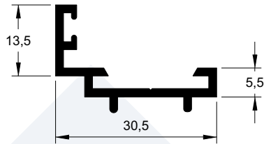
ES25-548 0,283 kg/m
