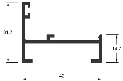
Y-351 0,440 kg/m
