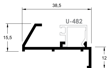
Z-063 0,325 kg/m
