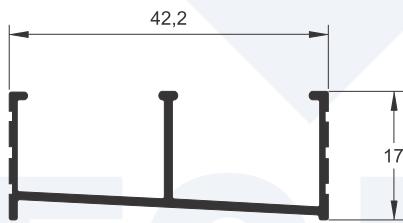
E-256 0,234 kg/m
