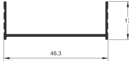
U-1245 0,183 kg/m
