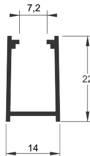
BXL-087 0,168 kg/m
