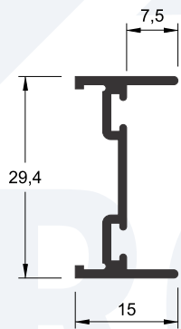
I-105 0,263 kg/m
