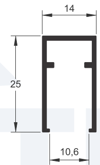
U-1056 0,187 kg/m
