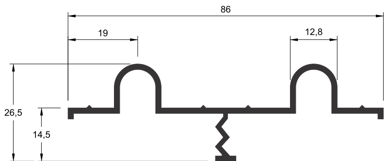
E-365 0,656 kg/m
