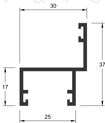
Y-126 0,260 kg/m
