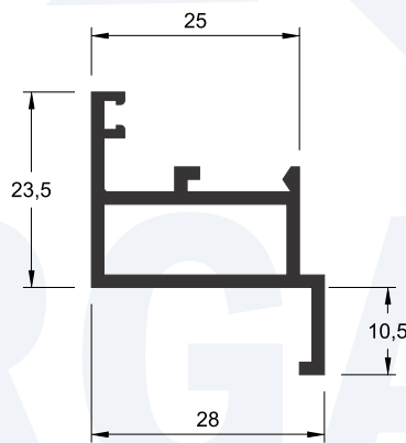
P-166 0,425 kg/m
