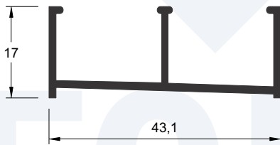
E-117 0,290 kg/m
