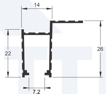
BX-091 0,200 kg/m
