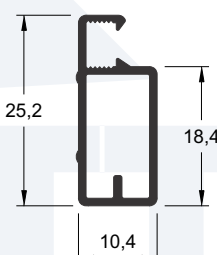
P-027 0,198 kg/m
