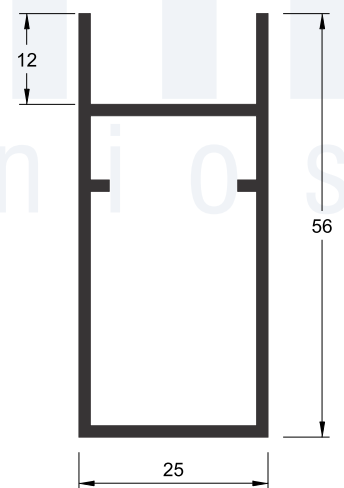
A-194 0,653 kg/m
