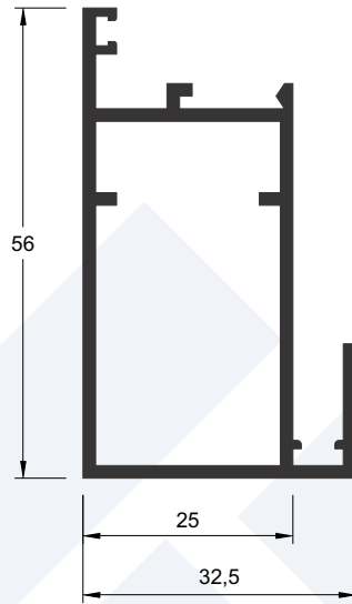
P-370 0,745 kg/m
