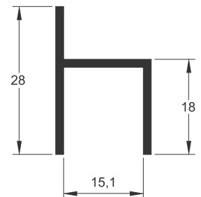
Y-107 0,212 kg/m
