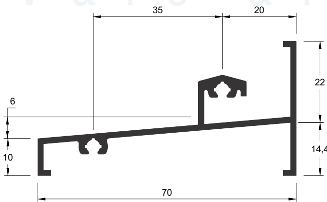
Z-174 0,726 kg/m
