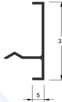
RA-007 0,156 kg/m
