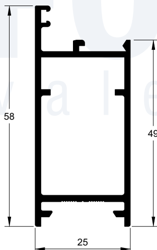
P-414 0,699 kg/m
