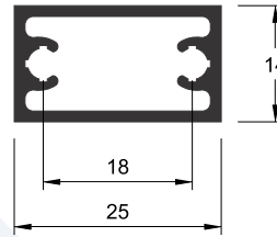
D-082 0,356 kg/m
