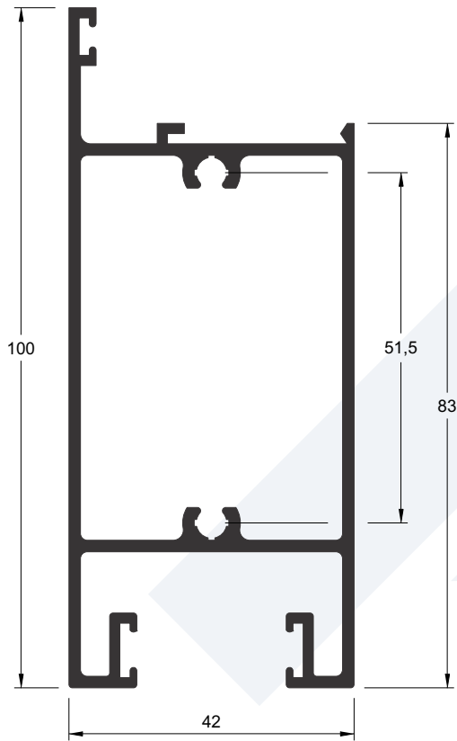
A-103 1,545 kg/m
