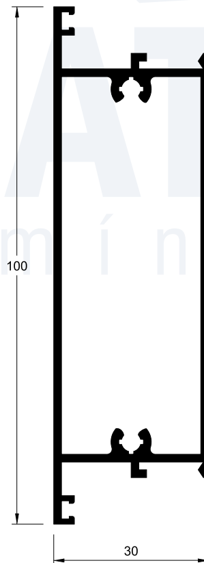
P-165 1,244 kg/m
