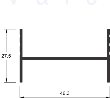
I-155 0,390 kg/m
