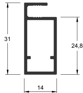
TM 1434 0,295 kg/m
