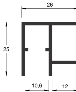
Y-105 0,222 kg/m
