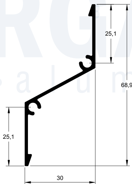
VZ-060 0,397 kg/m
