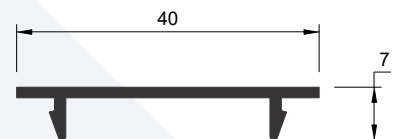
U-531 0,170 kg/m
