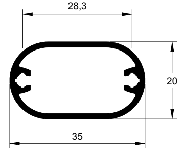
CG-087G 0,427 kg/m
