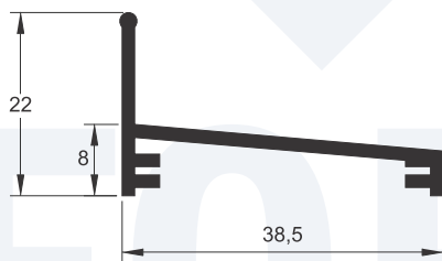
BXL-089 0,257 kg/m
