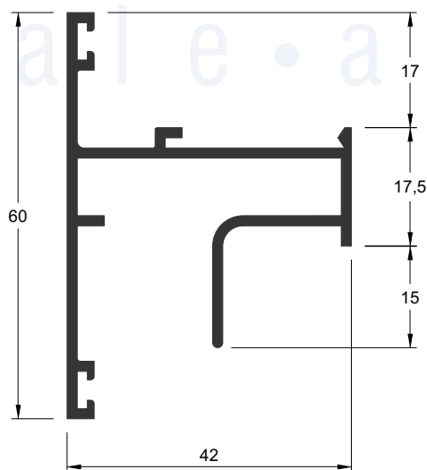
Y-273 0,705 kg/m
