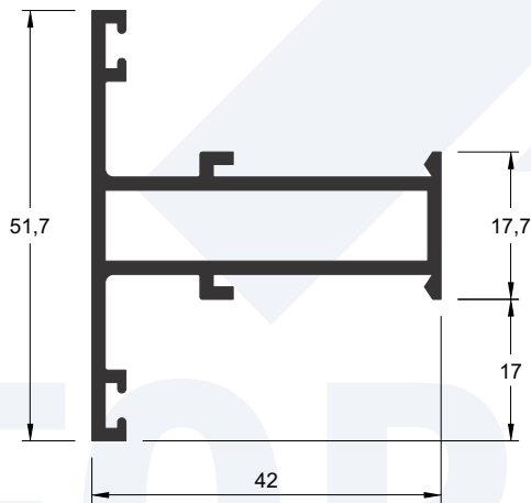
P-192 0,730 kg/m
