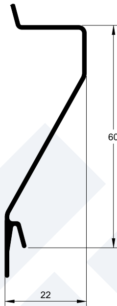
Z-203 0,325 kg/m
