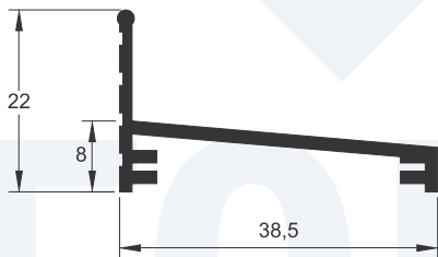
BX-089 0,251 kg/m
