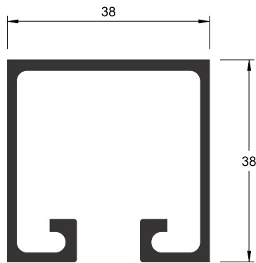
U-990 0,653 kg/m
