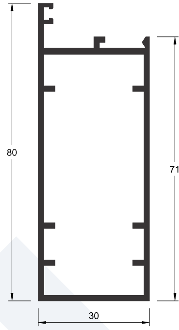
P-358 0,973 kg/m
