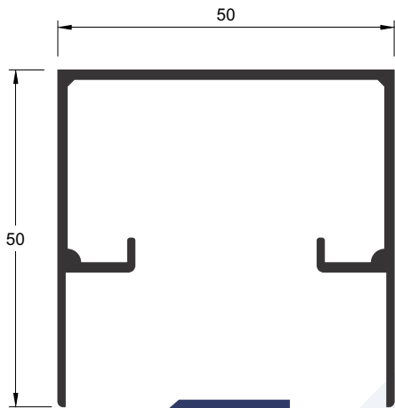
U-1242 0,600 kg/m
