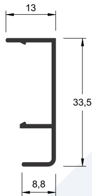
RA-130 0,166 kg/m
