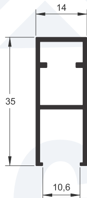
A-022 0,297 kg/m
