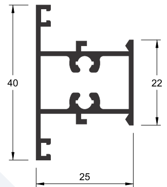
P-153 0,604 kg/m
