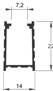
BX-087 0,154 kg/m
