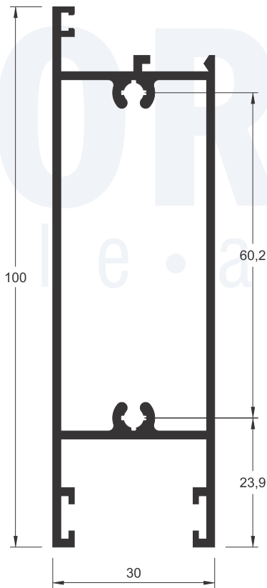
A-081 1,300 kg/m
