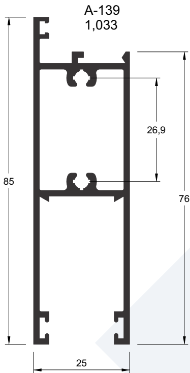
A-139 1,033 kg/m
