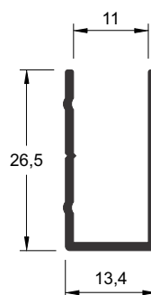
TM 2070 0,208 kg/m
