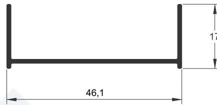
U-1244 0,240 kg/m
