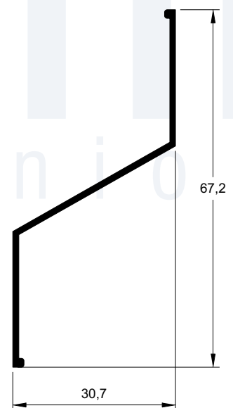
VZ-063 0,263 kg/m
