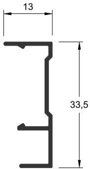
RA-111 0,173 kg/m
