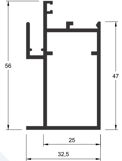
P-371 0,775 kg/m
