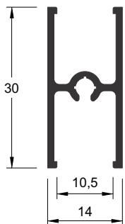
I-334 0,235 kg/m
