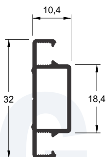
TM 1858 0,214 kg/m
