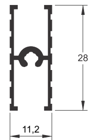
BX-090 0,208 kg/m
