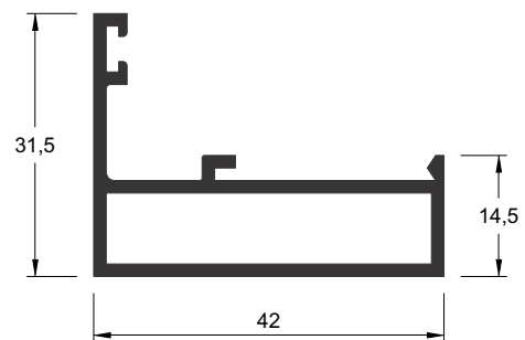
P-253 0,595 kg/m
