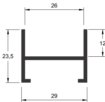
I-090 0,300 kg/m
