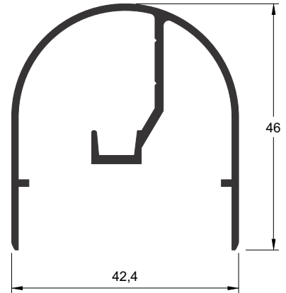
BXL-3918 0,506 kg/m
