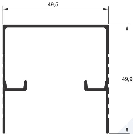
U-1243 0,534 kg/m
