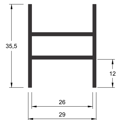
A-034 0,500 kg/m
