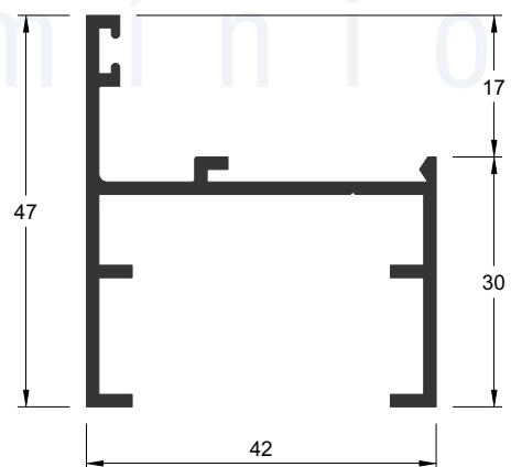
Y-271 0,610 kg/m
