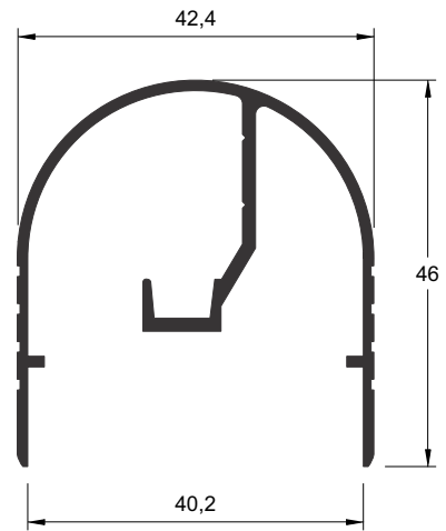
BX-140 0,504 kg/m
