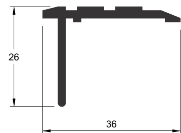
RA-029 0,369 kg/m
