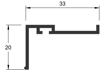
L-387 0,220 kg/m
