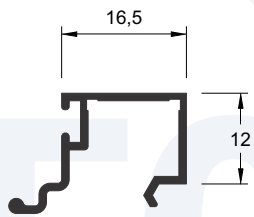
U-874 0,163 kg/m
