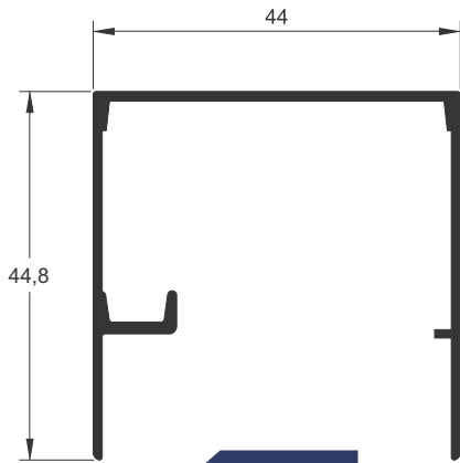
BXL-097 0,505 kg/m
