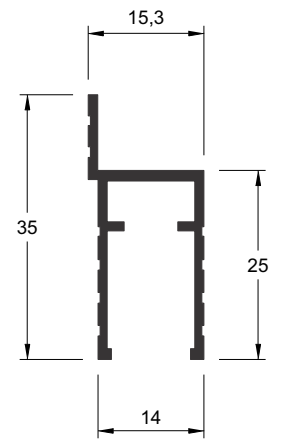
Y-310 0,243 kg/m
