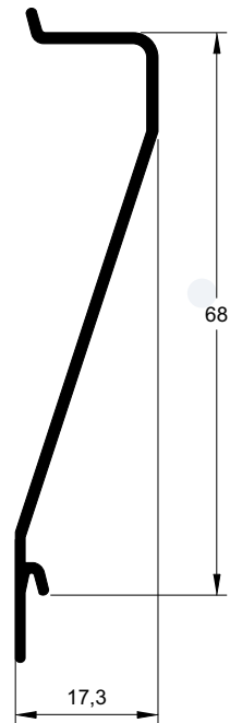
VA-017 0,266 kg/m
