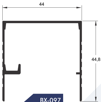
BX-097 0,495 kg/m
