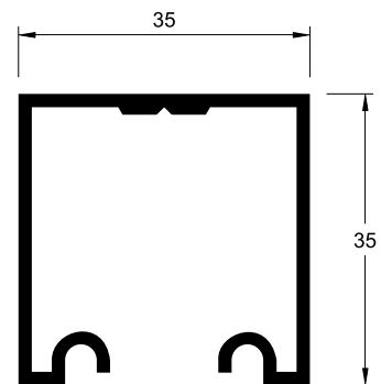
U-1098 0,494 kg/m
