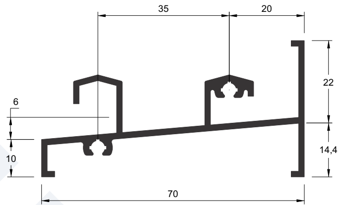
Z-176 0,854 kg/m
