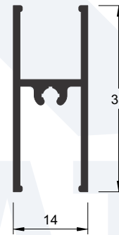
I-083 0,300 kg/m
